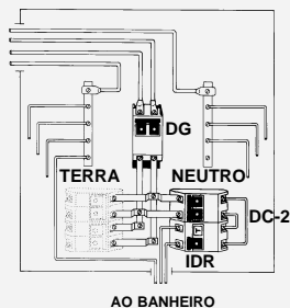
(A) FASE-FASE
